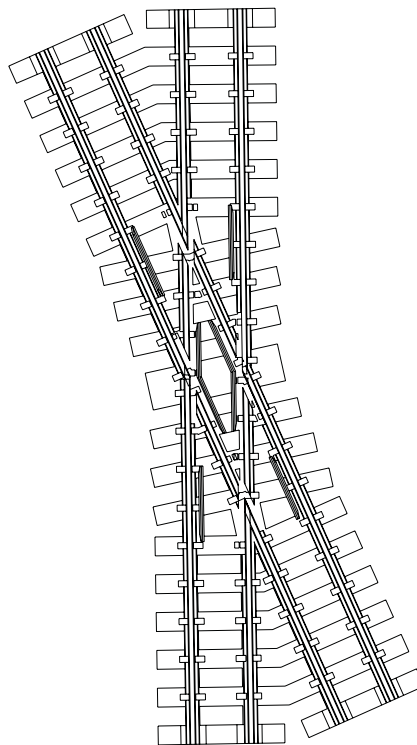
Kreuzung TTe 97,5 mm lang Profilh.2,07mm 25° Bestell.Nr. 50927
